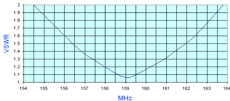
VSWR
